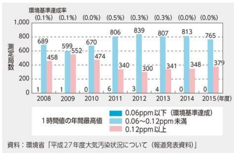
図 2. 光化学オキシダントの環境基準の達成状況
