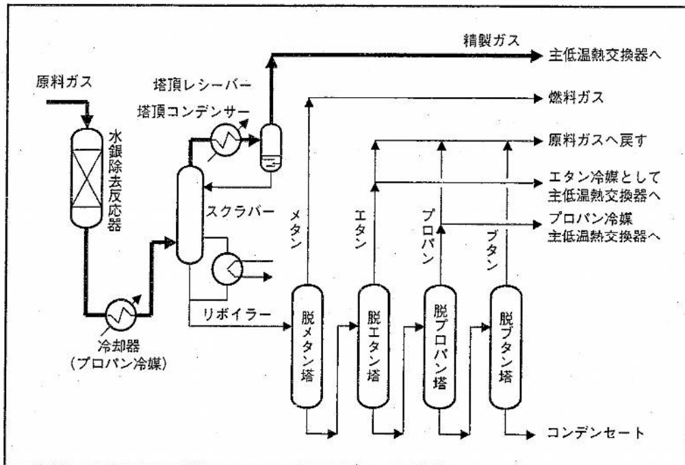
図 5. 炭化水素除去プロセス
