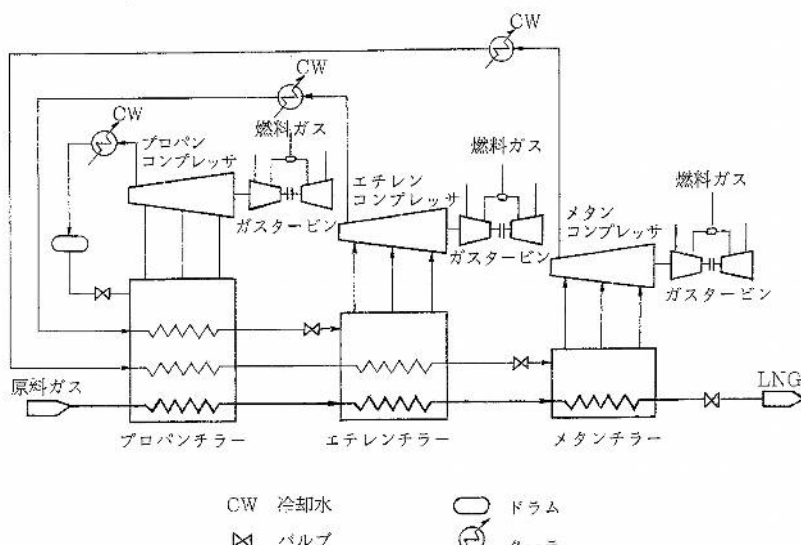
図 6. 多元冷媒カスケード方式液化プロセス
