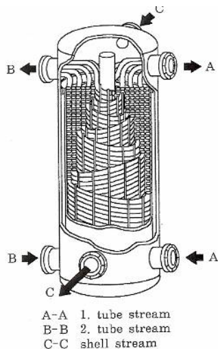
図8. ハンプソン式熱交換機
