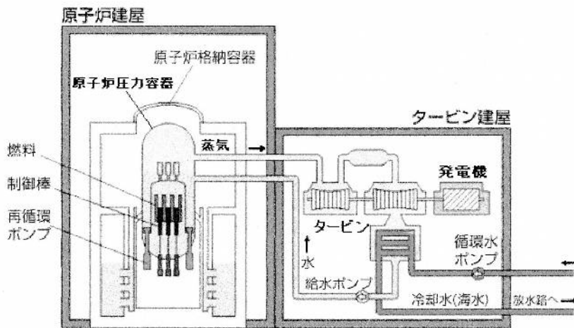
図 5. 原子力発電所の原子炉建屋とタービン建屋
