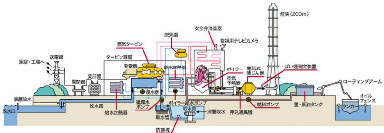
図2. 汽力発電所（石油燃料）の設備構成（九州電力川内発電所）出典：九州電力 HP
