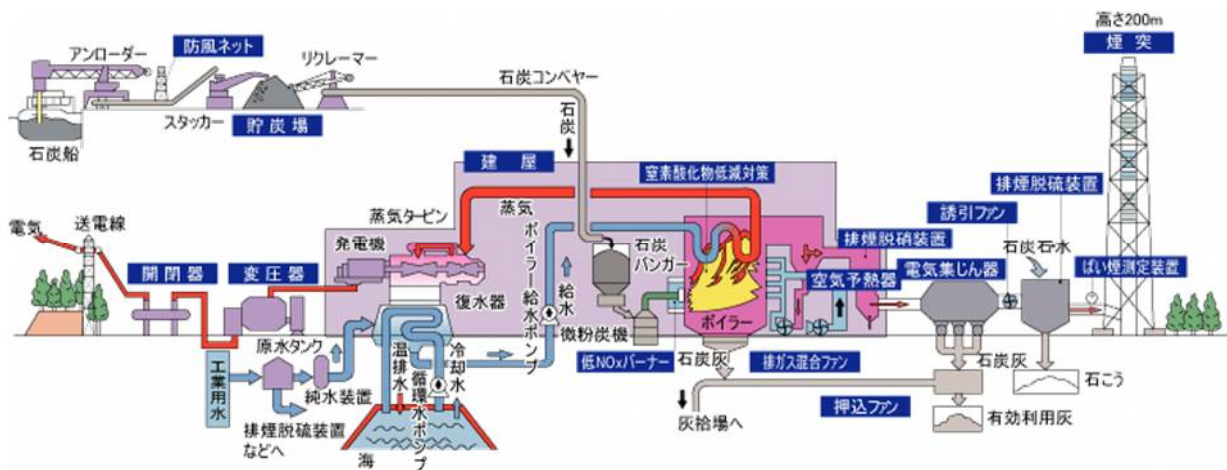
図 1. 汽力発電所（石炭燃料）の設備構成（九州電力苓北発電所） 出典：九州電力 HP
