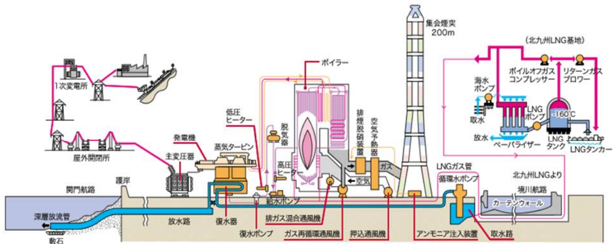
図 3. 汽力発電所（天然ガス燃料）の設備構成（九州電力新小倉発電所）出典：九州電力 HP
