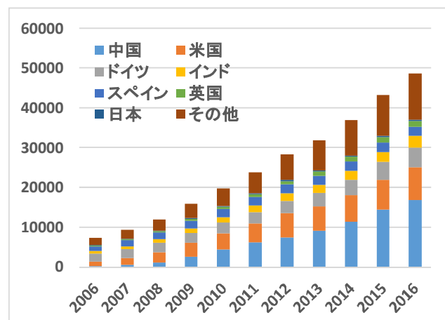
図 9. 風力発電の発電容量推移（万 kW）
